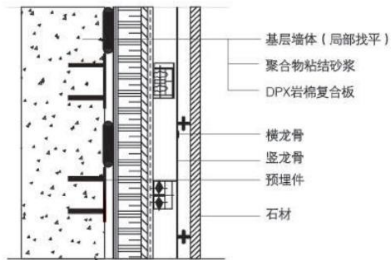
石材幕墙保温构造示意图
